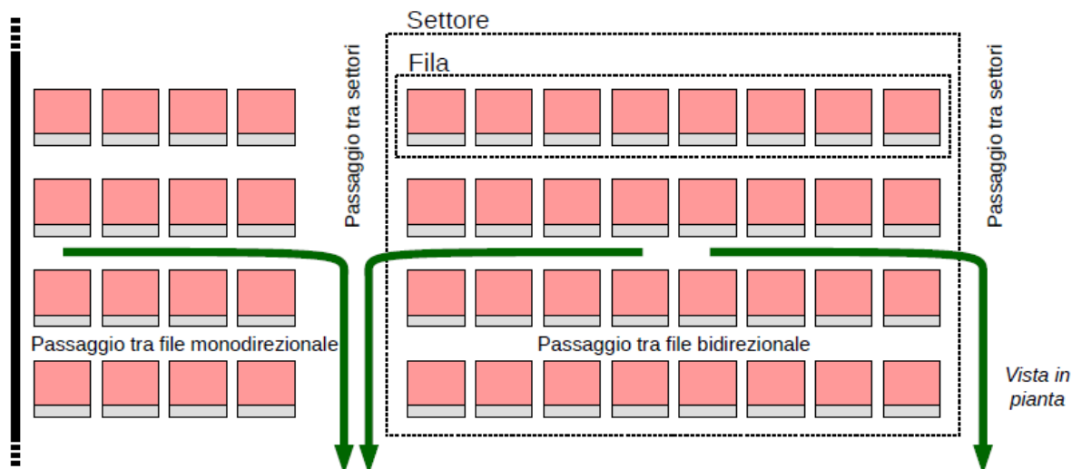
Illustrazione S.4-3 del codice di prevenzione incendi: Disposizione dei posti a sedere in settori e file
